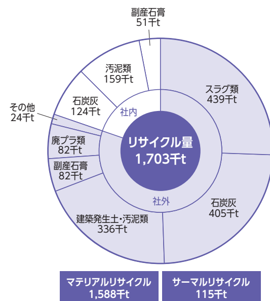
セメント製造工程における 廃棄物・副産物使用量 (2022年度)
